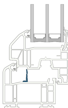
BOUCLIER THERMIQUE
